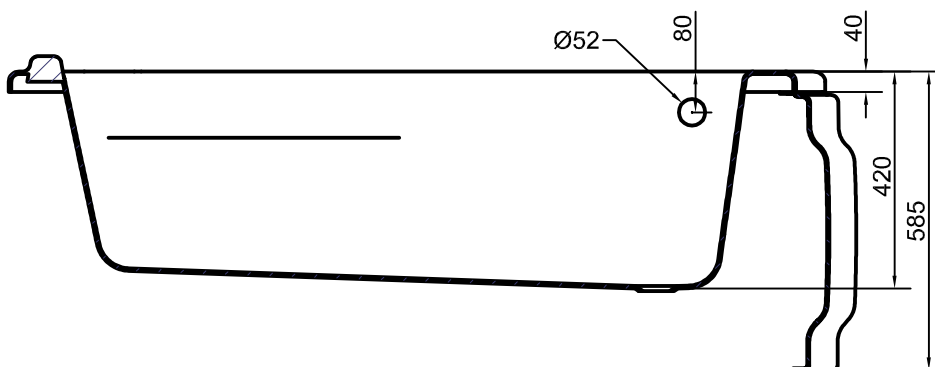
A-A (1 : 10)
