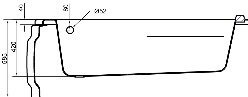
A-A ( 1 : 10 )
